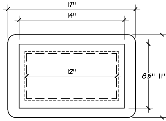
DV140-6x12
