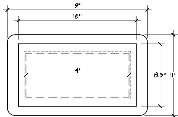
DV140-6x14
