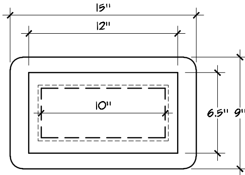
DV140-4x10
