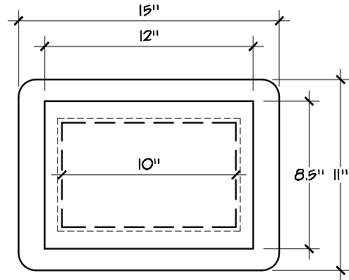
DV140-6x10
